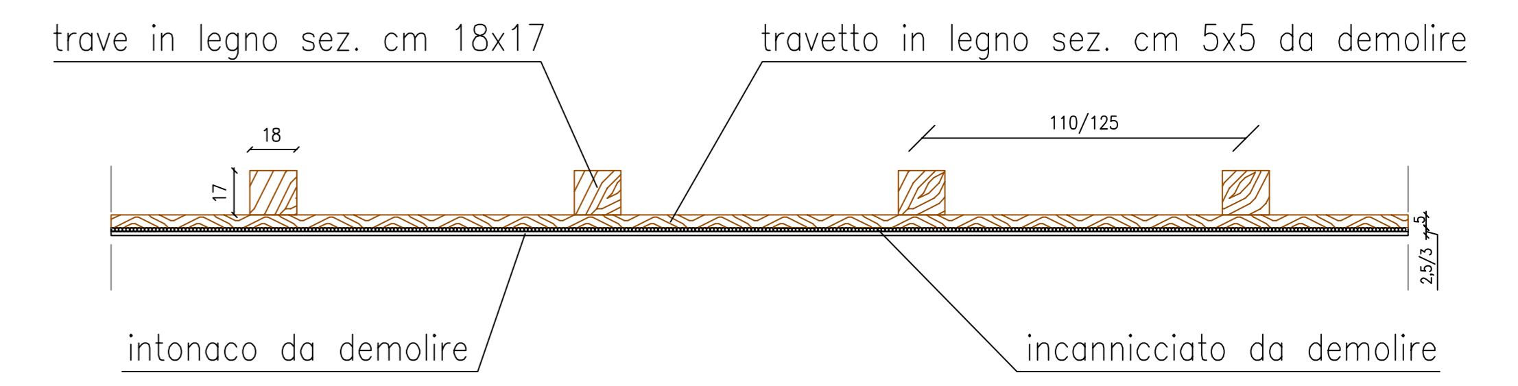
STATO DI FATTO scala: 1:10
