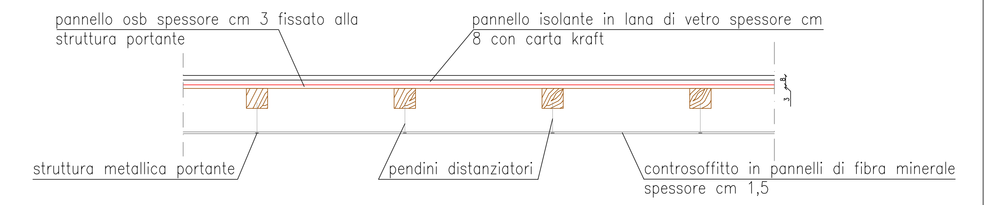
STATO DI PROGETTO scala: 1:10
